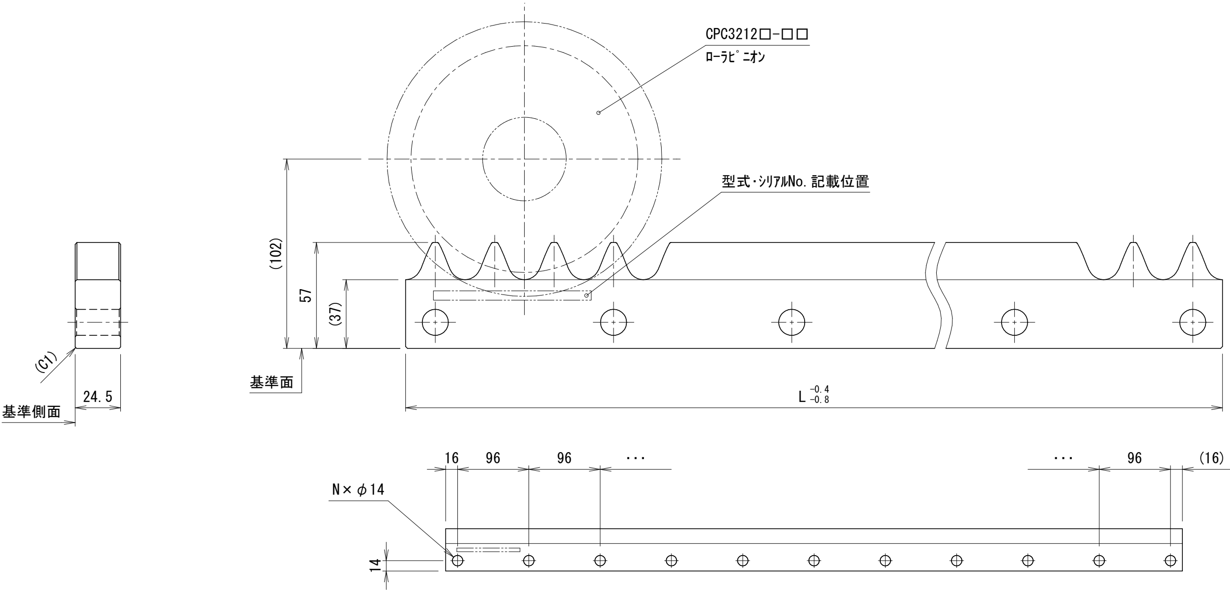
全体図 (1:5)
